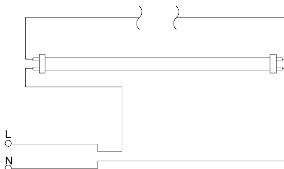
Схема подключения LED-лампы
