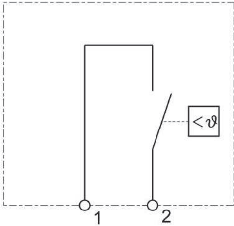
Электрическая схема
