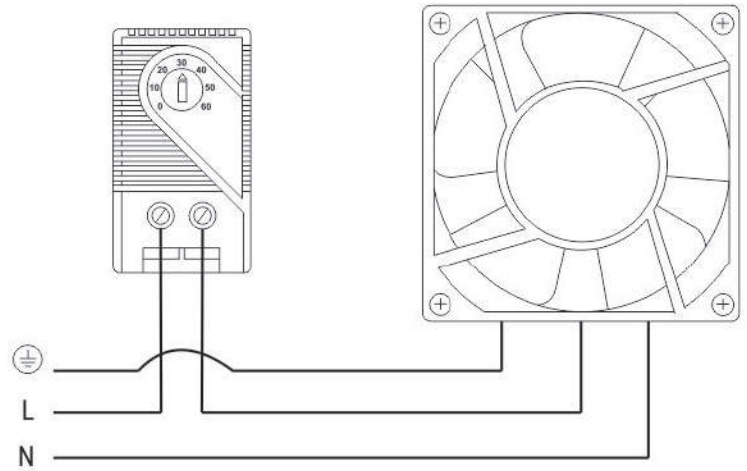
Пример подключения
